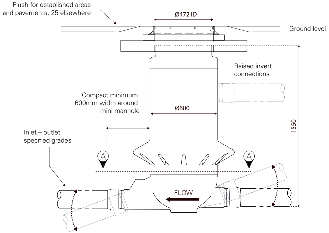
FIG. 3 Side elevation
