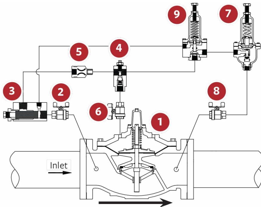
FIG. 2 Schematic A-0332C
